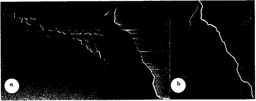
Abb. 8: Fotografie von Blitzen: a) mit einer Hochgeschwindigkeitskamera b) mit normaler Kamera [n. [11]]
