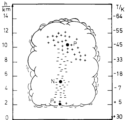
Abb. 1: Ladungsverteilung in einer Gewitterwolke
