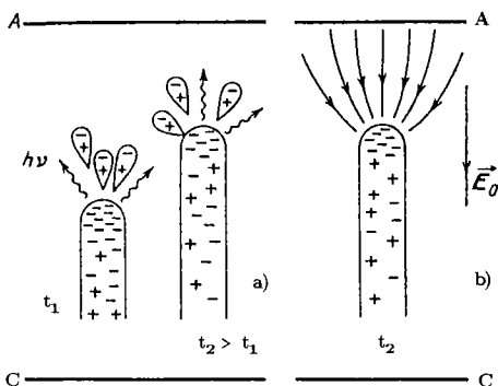
Abb. 6: a) Sekundärlawinen und Photonen [9] b) E-Feld in der Nähe des Kopfes [9]
