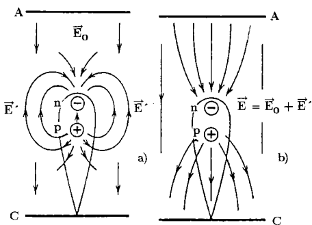
Abb. 5: Elektronenlawine u. äußeres Feld (n. [9]) n,p: Raumladungszentren
