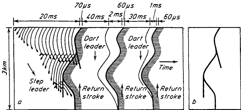
Abb. 9: a) Skizze eines mit einer Boy's-Kamera auf bewegtem Film aufgenommenen Blitzes. b) Skizze des Blitzes bei einer normalen Kameraaufnahme (n. [9]).
