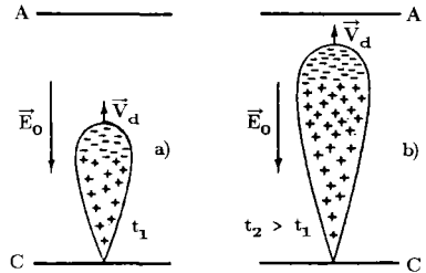
Abb. 3: Gestalt und Ladungsverteilung in einer Elektronenlawine (n. [9])
