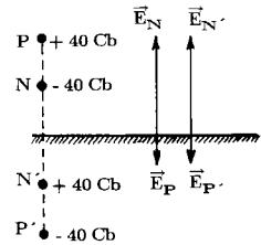
Abb. 2: Erläuterung i. Text
